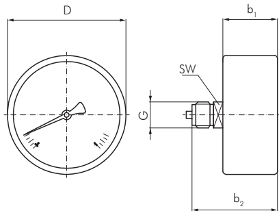
Manometer
