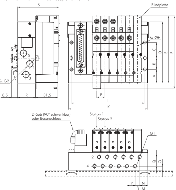
Ventilterminal mit Anschlussplattenventilen
