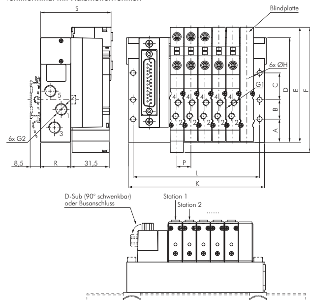
Ventilterminal mit Halbmuffenventilen
