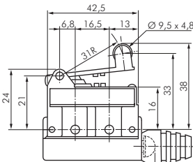
Zeichnung 2
