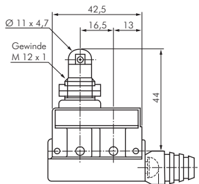
Zeichnung 5
