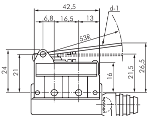
Zeichnung 1
