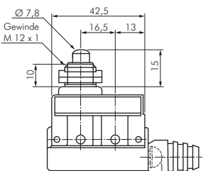
Zeichnung 4
