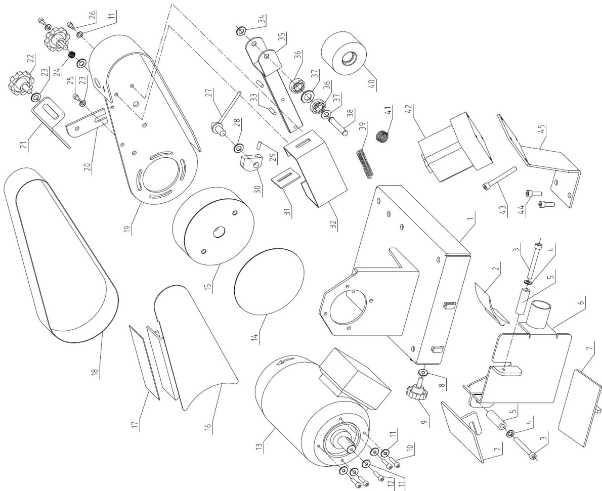
Abb. / Fig. 1: Ersatzteilzeichnung 1/ Spare parts drawing 1
