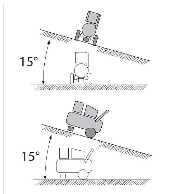
Abb. 5: Kompressor aufstellen
