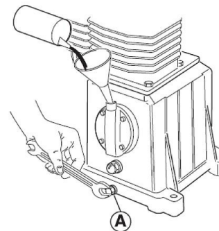
Abb. 18: Ölwechsel
