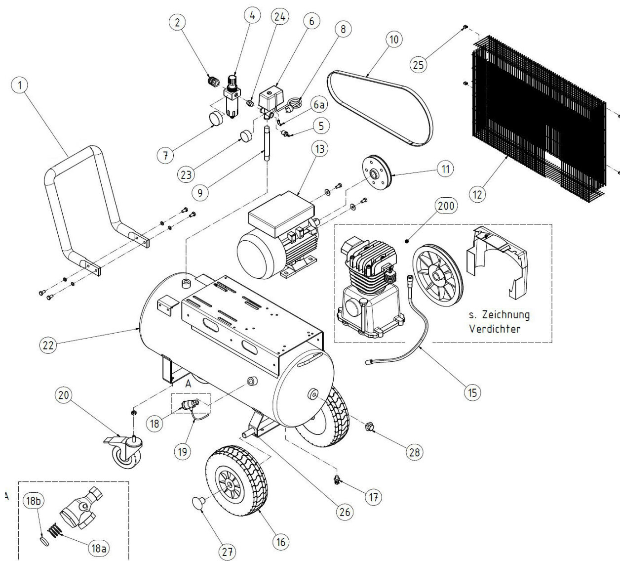
Abb. 25: Ersatzteile AIRSTAR 503/50
