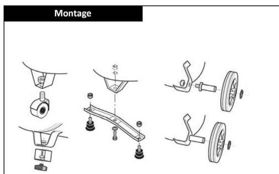
Abb. 3: Räder-Montage
