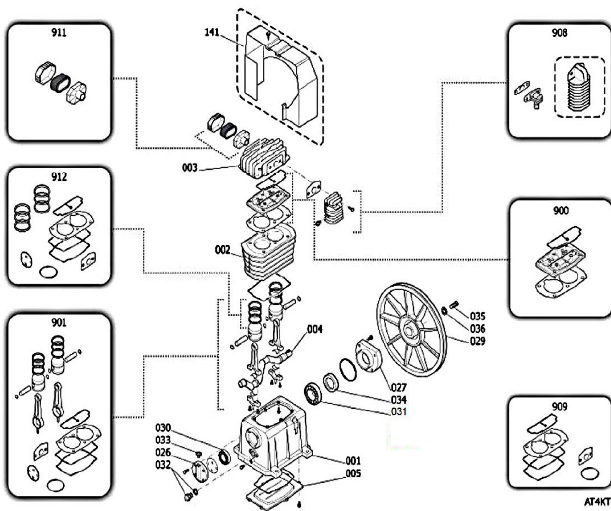
Abb. 27: Verdichter MK 113
