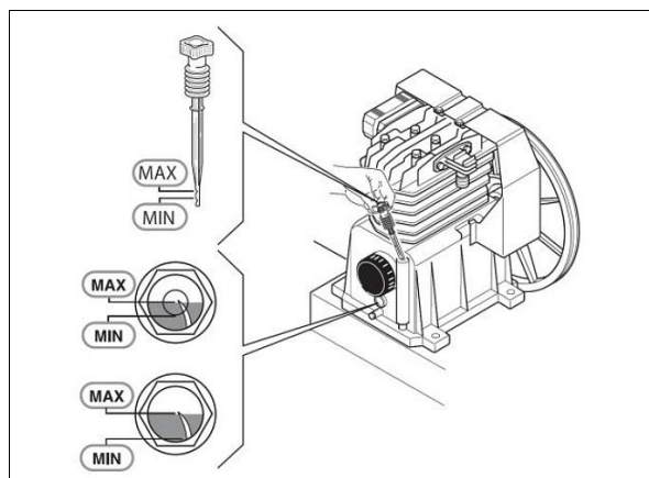
Abb. 4: Ölstand-Anzeige
