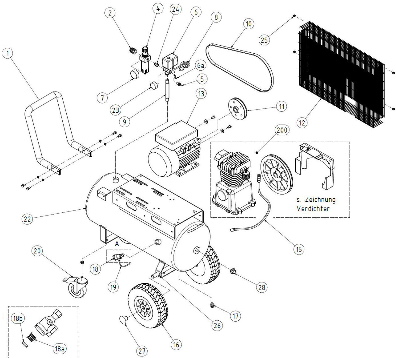
Abb. 23: Ersatzteile AIRSTAR 401/50, 401/100, 403/50 und 403/100
