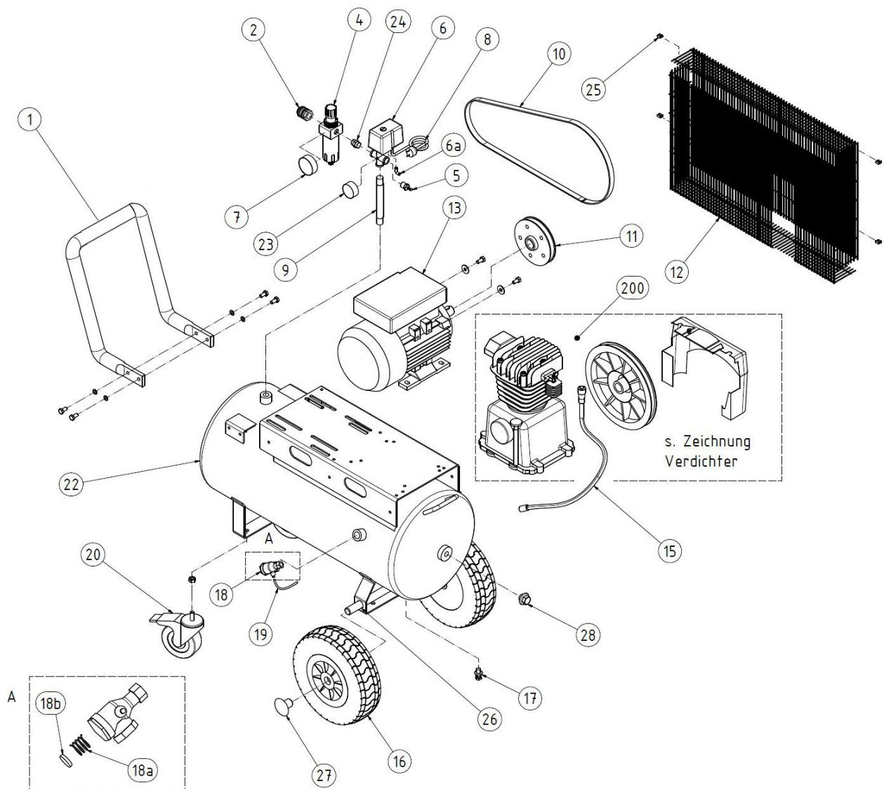
Abb. 26: Ersatzteile AIRSTAR 503/100
