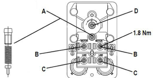
Abb. 13: Druckschalter MDR 1
