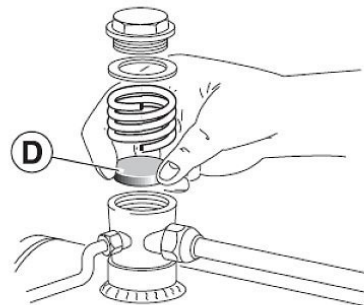
Abb. 20: Dichtelement im Rückschlagventil
