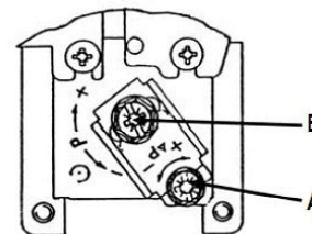
Abb. 15: Druckschalter MDR 3
