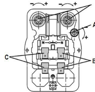
Abb. 14: Druckschalter MDR 2
