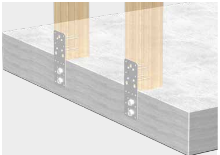
Montaje sencillo de dos elementos de madera sobre una placa de hormigón con los conectores planos pesados.
