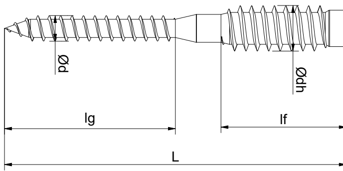
Vista lateral
