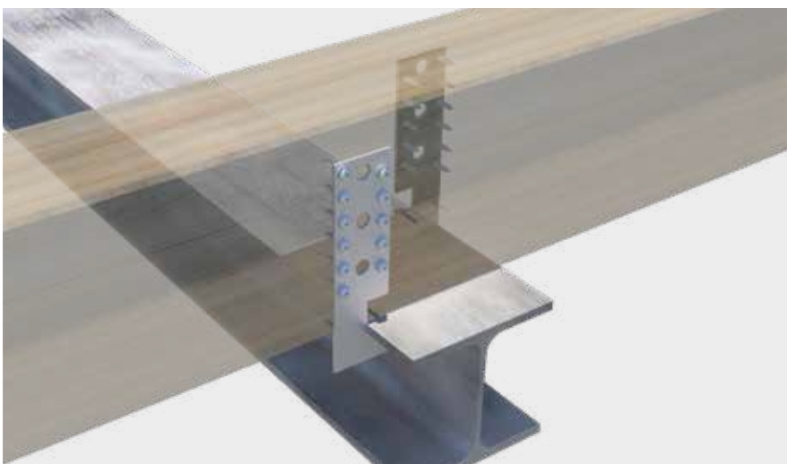
Anclaje para perfiles en T con un perfil en T
