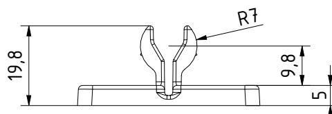
Вид сбоку
