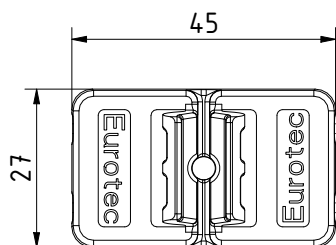
Вид сверху
