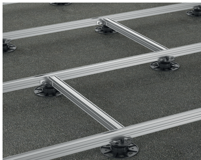
Stopa przestawna BASE z aluminiowym profilem systemowym EVO Light
