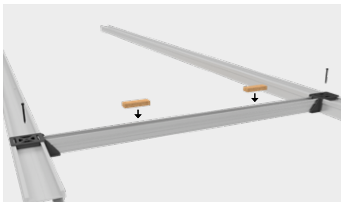
Widok rozstrzelony poszczególnych części konstrukcyjnych
