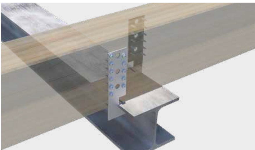
Ancoraggio supporto a T abbinato a un supporto a T.
