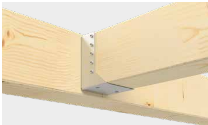
Collegamento di due travi in legno mediante la staffa ali interne.
