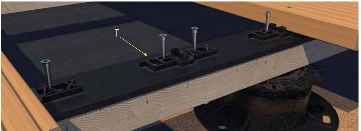
Il distanziatore Tenax (T) su una sottostruttura in legno
