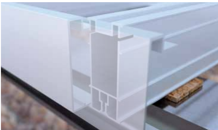
Esempio di applicazione TERRA Profilo di rivestimento H85
