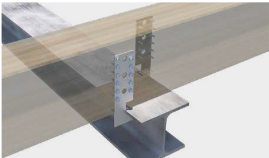
Ancrage de poutrelle en T combiné à une poutrelle en T.
