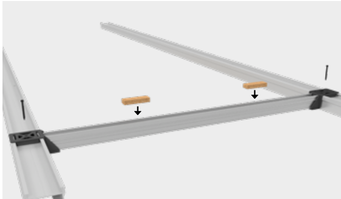
Vue éclatée des différents composants
