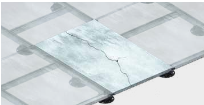
Risque accru de rupture de panneaux en raison de l'absence de profilés supports
