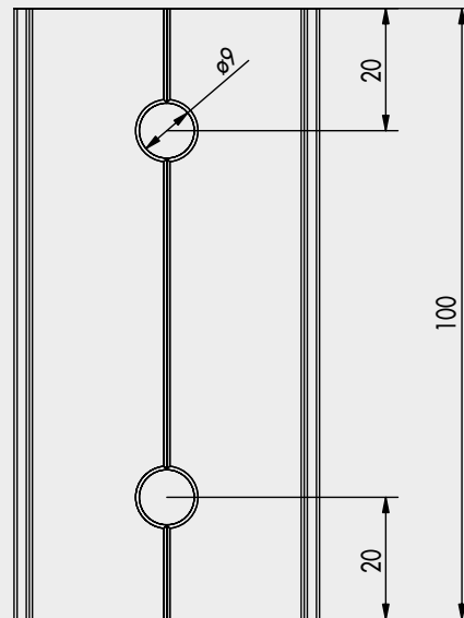
Seitenansicht
