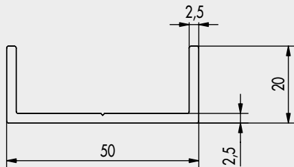
Vorderansicht
