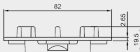
Seitenansicht
