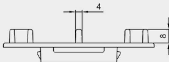
Seitenansicht
