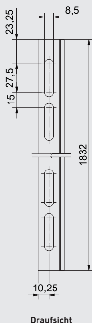
Draufsicht
