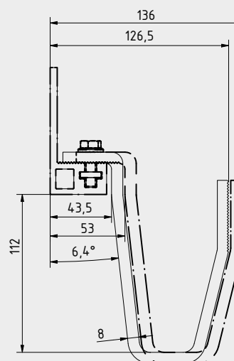
Seitenansicht
