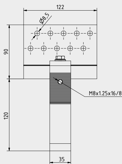
Vorderansicht
