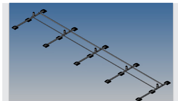
SCHRITT 5: LASTVERTEILPLATTEN UND DACHSCHUTZKORK
