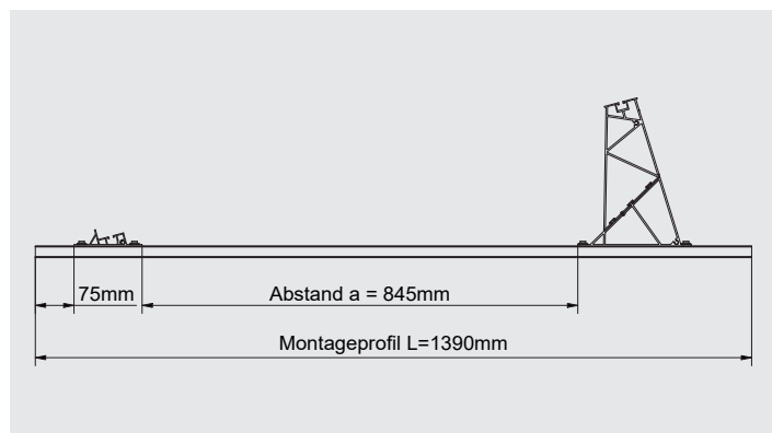
SÜDAUSRICHTUNG 15°: MAßE DER STRÄNGE (L2) DER LETZTEN REIHE
