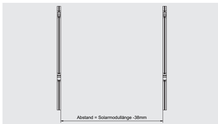
SCHRITT 2: VORMONTIERTE STRÄNGE IM ABSTAND AUSLEGEN
