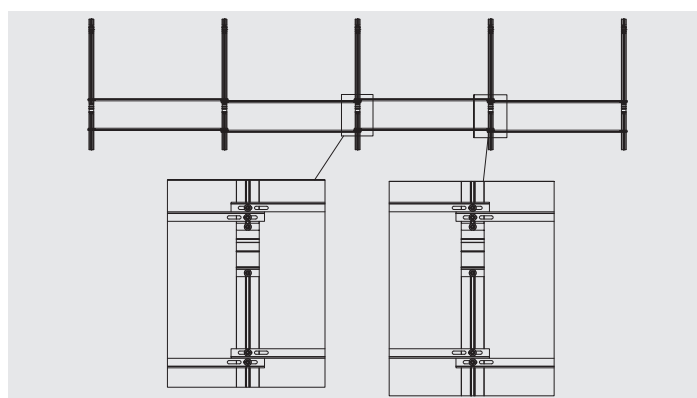
SCHRITT 4: UNTERKONSTRUKTION ERWEITERN
