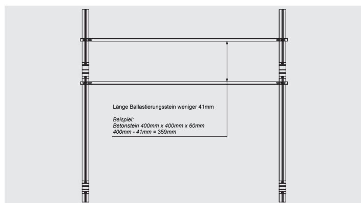
SCHRITT 3: BALLASTPROFILE BEFESTIGEN
