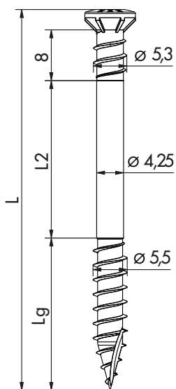
Seitenansicht
