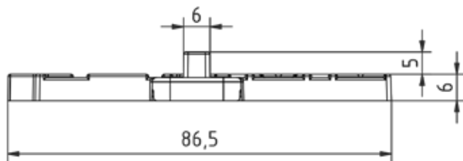
Seitenansicht
