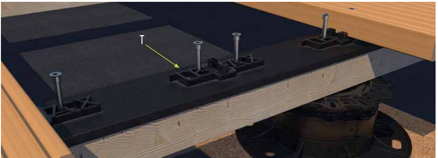
Der Tenax-Distanzhalter (T) auf einer Holzunterkonstruktion
