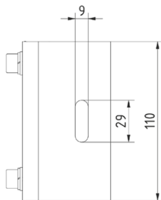
Draufsicht
