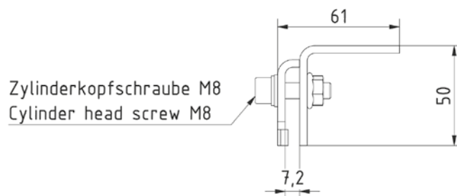
Seitenansicht
