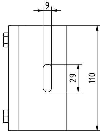
Draufsicht
