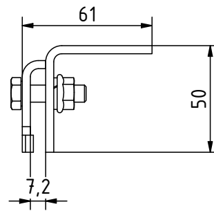
Seitenansicht
