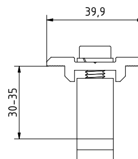
Vorderansicht, Endklemme
