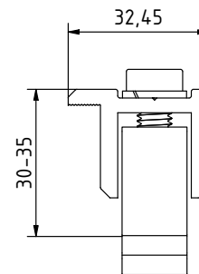
Vorderansicht, Endklemme
