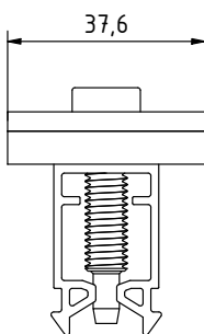
Seitenansicht, Endklemme
