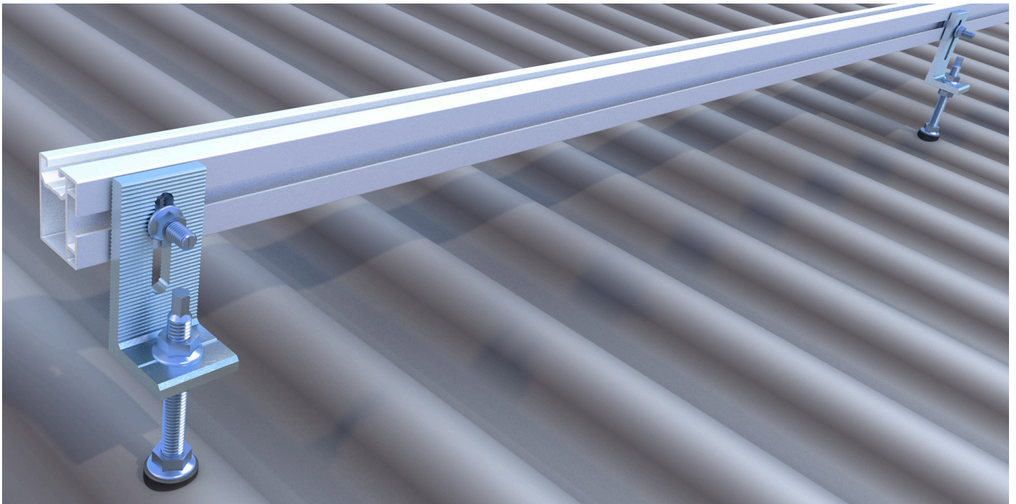
L-Adapter und Solarstockschraube zur Befestigung eines Montageprofils auf einem Wellblechdach
