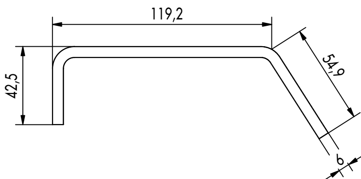
Seitenansicht
