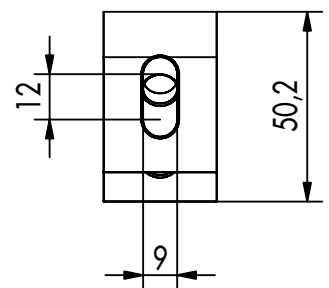
Vorderansicht
