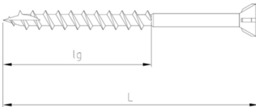
Seitenansicht
