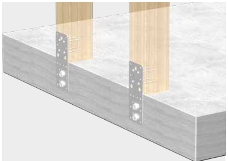
Einfache Montage von zwei Holzelementen auf einer Betonplatte durch die Flachverbinder schwer.
