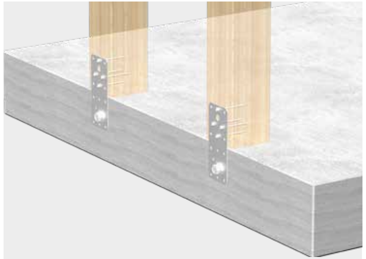
Einfache Montage von zwei Holzelementen auf einer Betonplatte durch die Flachverbinder leicht.
