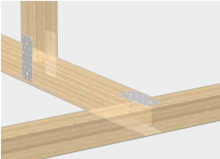
Schnelle Verbindung mehrerer Holzelemente durch die Flachverbinder leicht.
