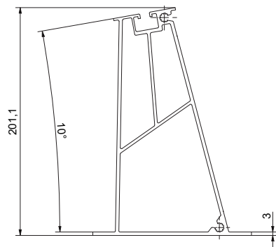
Seitenansicht 10°
