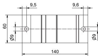
Draufsicht 10°
