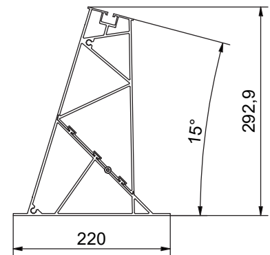
Seitenansicht 15°
