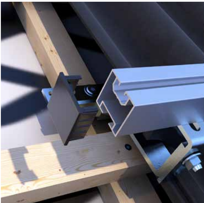
Endkappen im befestigten Zustand am Montageprofil Steildach und Steildach SLIM.
