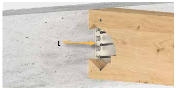
Der EST Stabdübel (E) in einer Holz-Aluminium-Verbindung.
