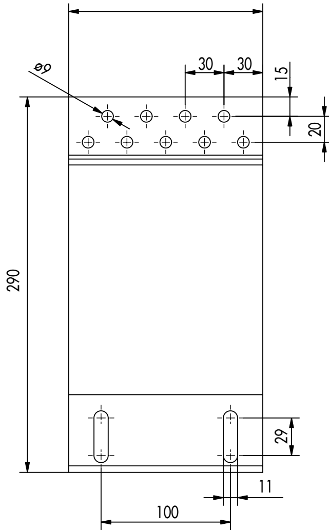
Vorderansicht
